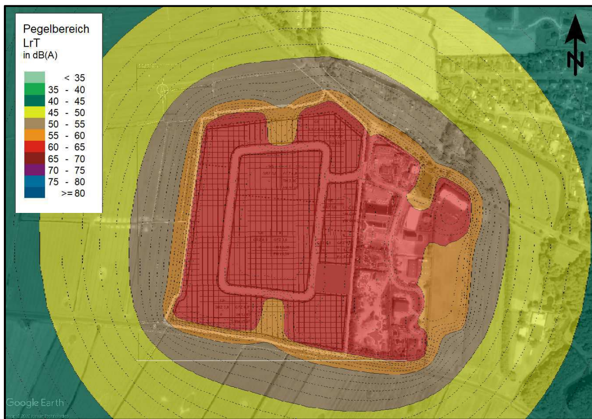
Abbildung 11: Rasterlärmkarte Gesamtbelastung, Tagbeurteilungszeitraum, h = 5,5 m
